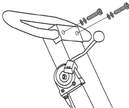
Рис. 4 Установка рабочей рукоятки PC1645RH
